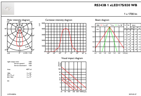
IFAS1_RS343B1xLED17S830WB
