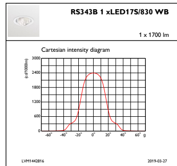
IFCC1_RS343B1xLED17S830WB
